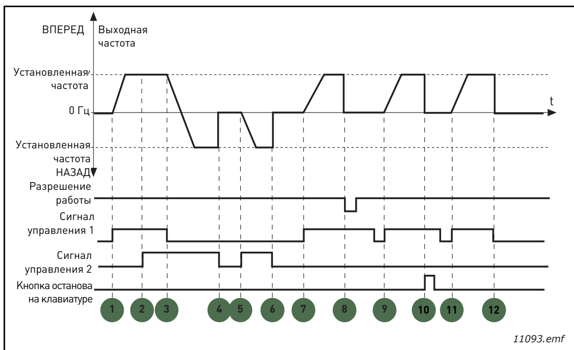
Рис. 21. Логика пуска/останова от платы ввода/вывода А = 2
